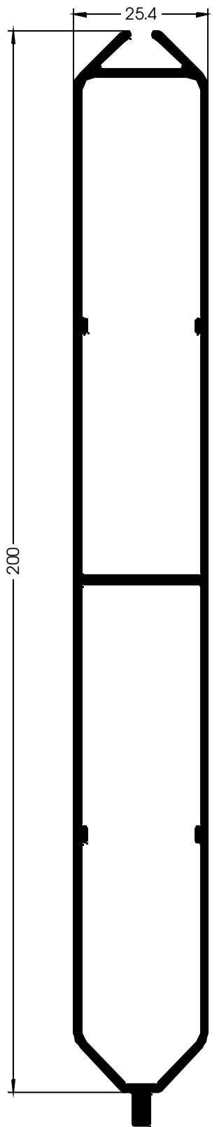
Ref. APT035 (*) LAMA BISELADA 200x25 (puertas)
