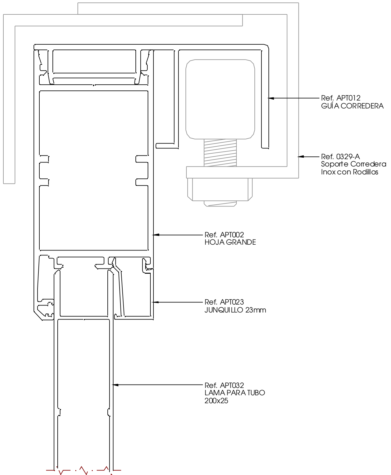
SECCIÓN VERTICAL ESCALA 1:1
