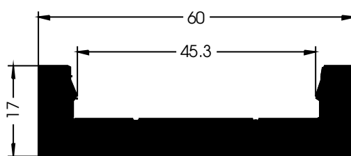
Ref. AP1718 SOPORTE SUJECCIÓN AL MOTOR
