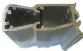
Ref. 0327-G27 Tope de Unión para Marco y Hoja Pequeña 27.5mm
